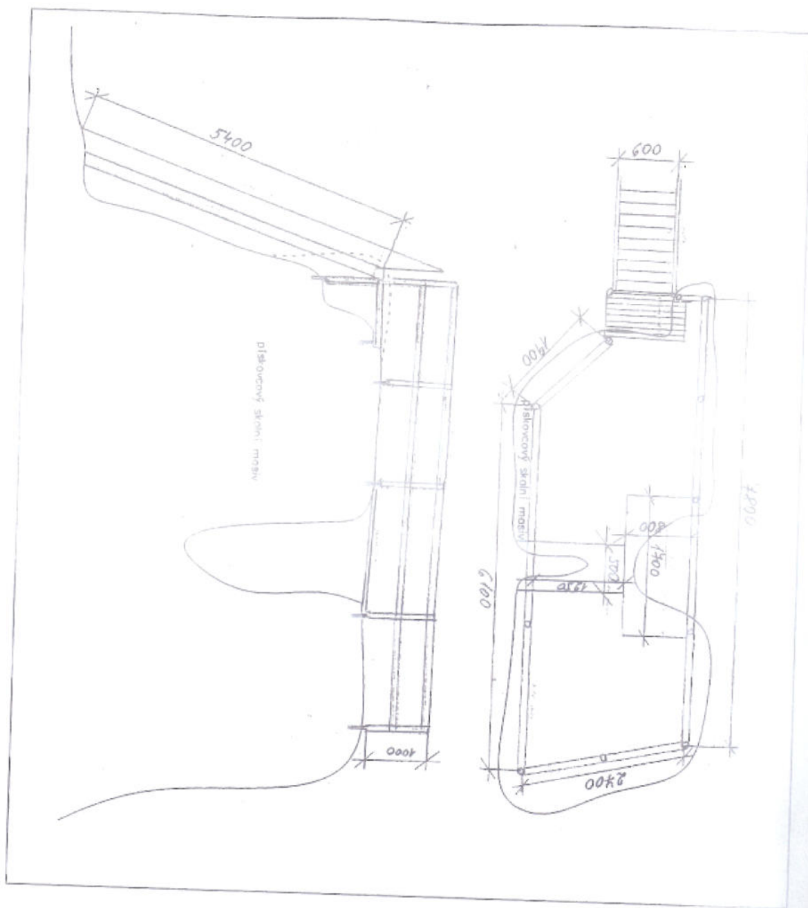
Situační náčrt
