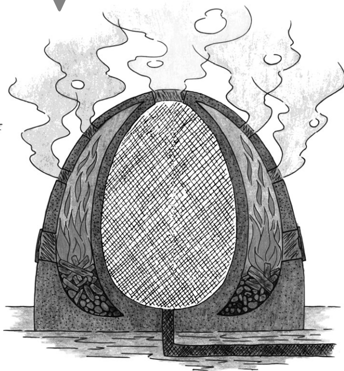
Průřez dehtářskou pecí
